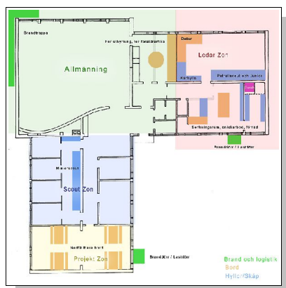
Så här såg första utkastet till ombyggnadsförslag ut våren 2004
